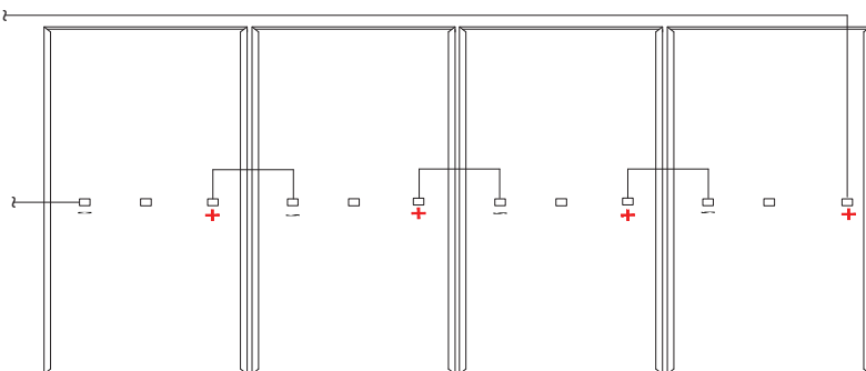
Conexión LeapFrog (Conexión de módulos en posición vertical)
