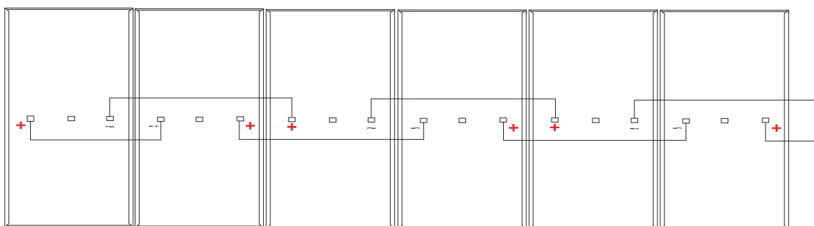
Conexión LeapFrog (Conexión de módulos en posición vertical)
