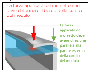
Figura 1 Forza applicata dal morsetto
