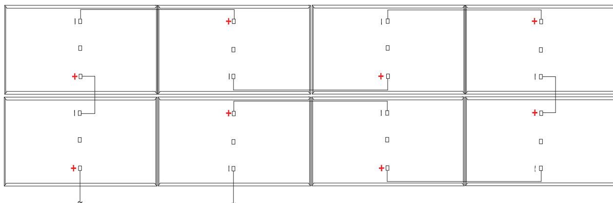
Conexión de los módulos en posición horizontal
